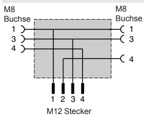
FTX CY1208
