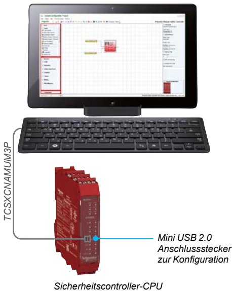
Sicherheitscontroller-CPU
