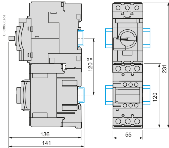
Montage vertikal (1)
