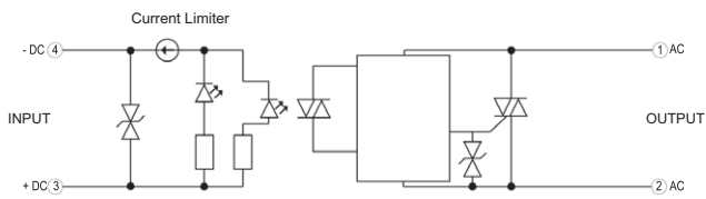
Contrôle 4-32 V DC série GN (Triac) - 10 A / 25 A (280 V AC )
