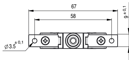
Plaques de montage PT avec trous 79556204
