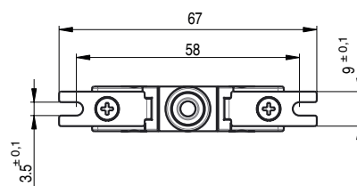
Plaques de montage PE avec encoches 79556205
