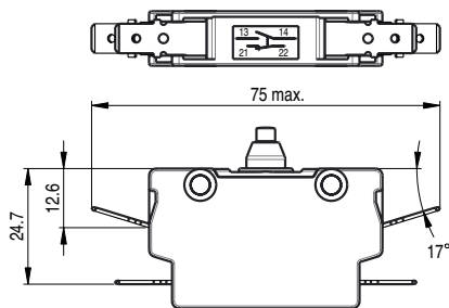
Vis W5/IP20 avec protection pince IP20
