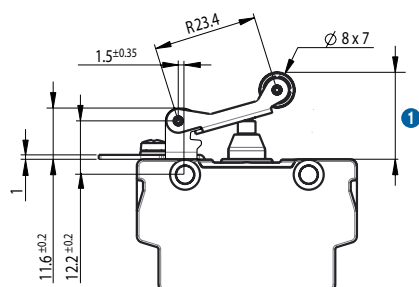
Levier à galet LG PE + plaques à encoches 79556203
