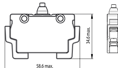
Couvercle de connexion à vis IP20 79556165
