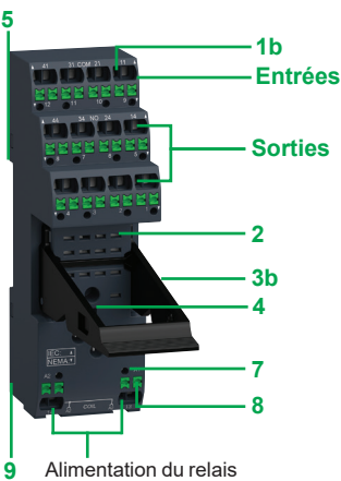
Embases avec contacts séparés
