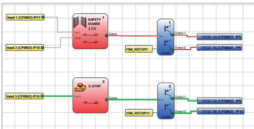
Visualisation graphique
